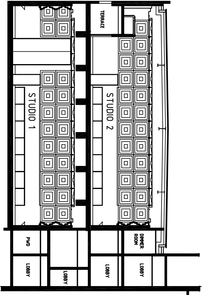
LONGITUDINAL SECTION
