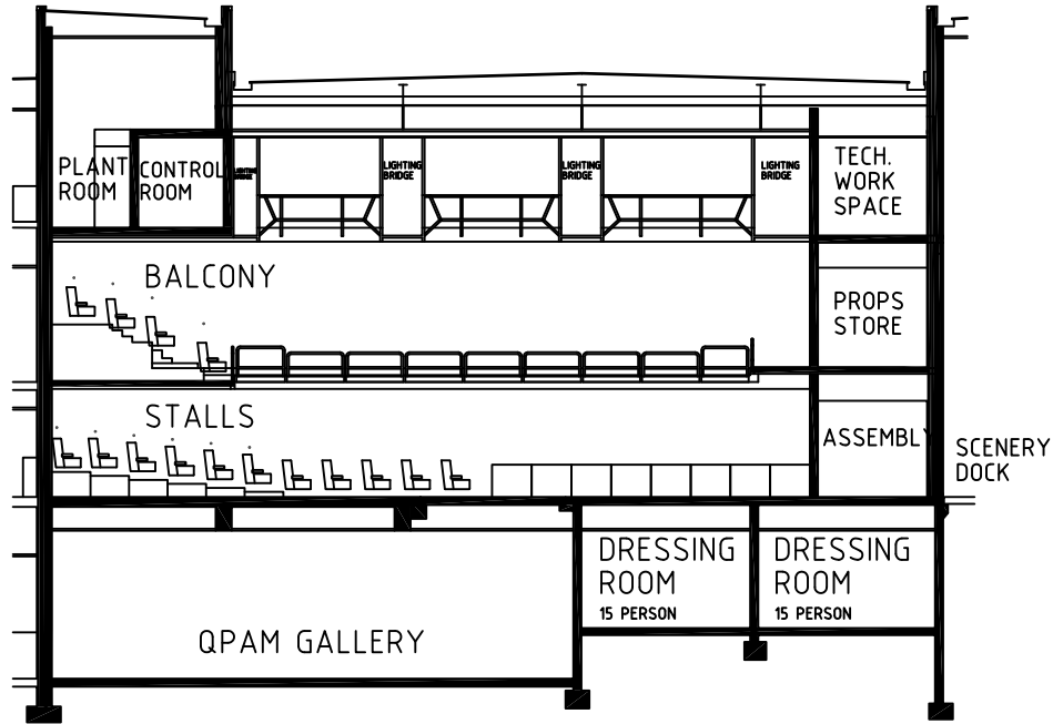
LONGITUDINAL SECTION
